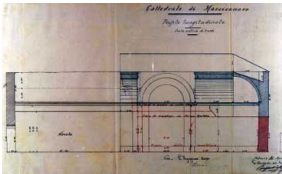
Fig. 6: Cattedrale di Marsiconuovo: Sezione della Chiesa allegata alla perizia dell'aiutante del Genio Civile Raffaele Pergola del 10 aprile 1888. Per constatare la parte di muratura eseguita e anche per avere un riferimento con quella che si sarebbe eseguita dopo, è stata rilevata una sezione della chiesa nella quale sono tracciati in rosso le parti di muratura eseguite a tutto agosto 1886, "... ed in linee azzurre la parte, che a mio giudizio, si può eseguire col fondo disponibile delle lire 14995,54 concesso dal Ministero.". ASPZ - PREFETTURA 1888-1892. Categ. 9, Titolo X: Culto.* (Foto E. Salinardi)
