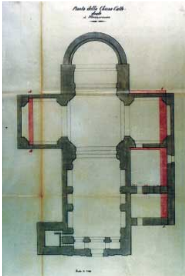
Fig. 7: Cattedrale di Marsiconuovo: Pianta della Chiesa allegata alla perizia dell'aiutante del Genio Civile Raffaele Pergola del 10 aprile 1888. La ricostruzione dei muri laterali del transetto risultano più corti di quelli originali: "... perché i due brani della crociera sono stati impiantati più brevi di quelli risultanti dalla planimetria e si arrestano alle linee AB e CD, tracciate in rosso ...". ASPZ - PREFETTURA 1888-1892. Categoria 9, Titolo X: Culto.* (Foto E. Salinardi)
